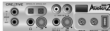
Модуль Sound Blaster Audigy 2 Drive
